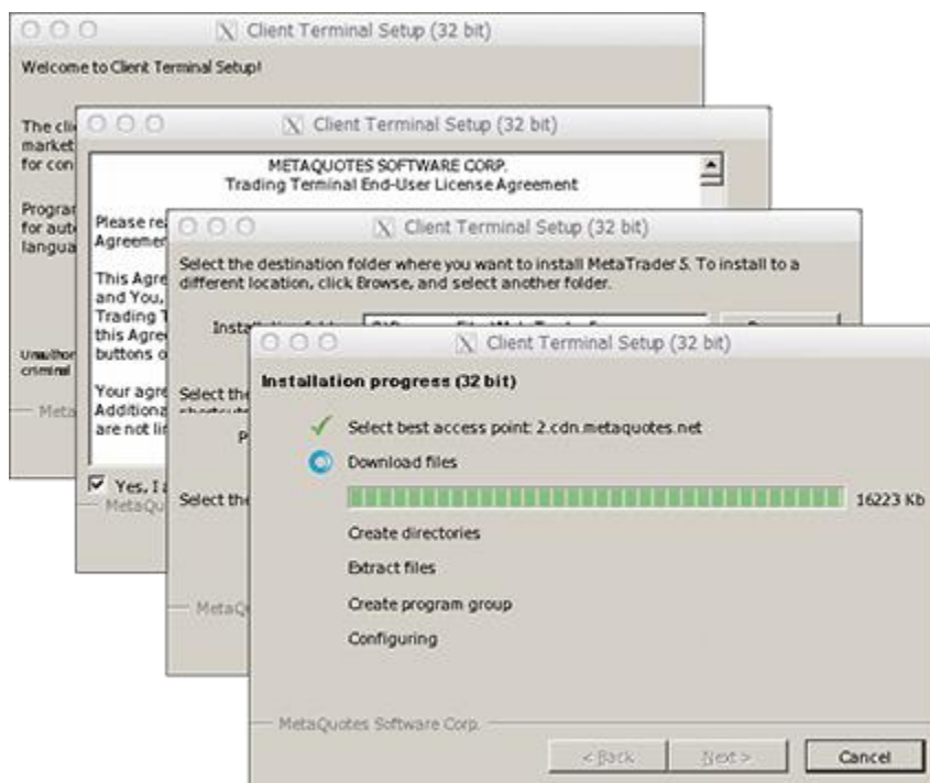
Obr. 14. Instalace terminálu
