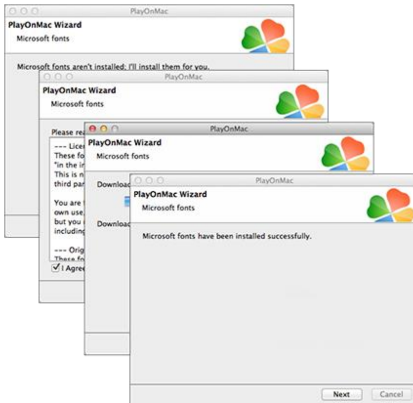
Obr. 8. Spuštění PlayOnMac
