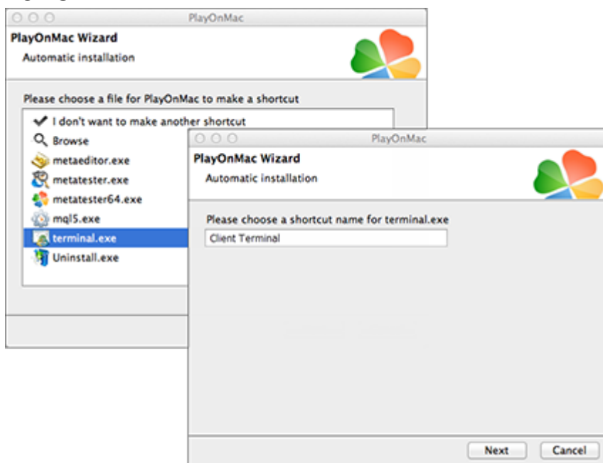
Obr. 15. Vytvoření zkratk
