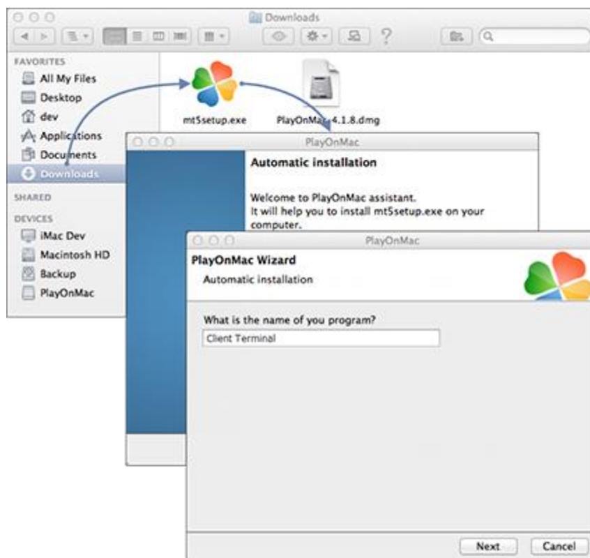
Obr. 13. Instalace terminálu
