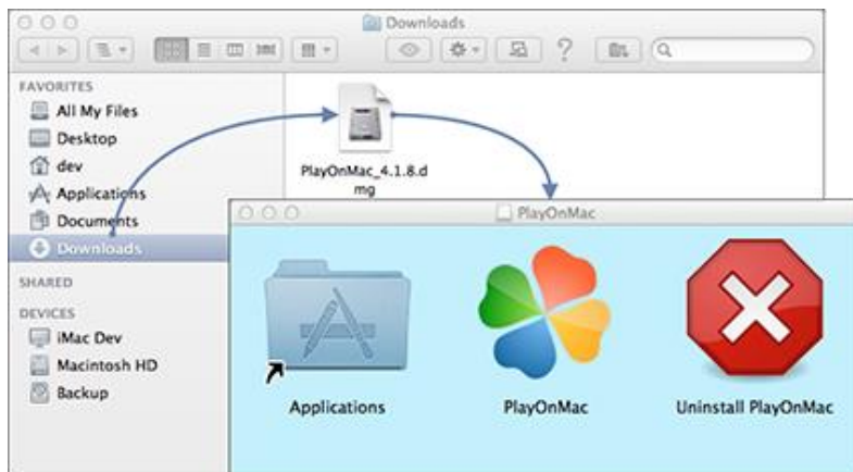
Obr. 2. Otevření DMG
