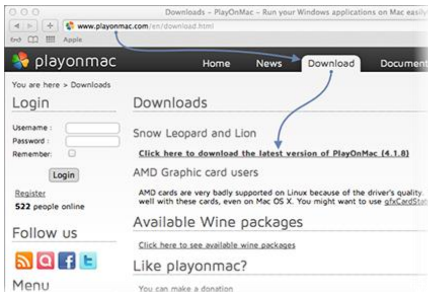
Obr. 1. Stažení PlayOnMac
